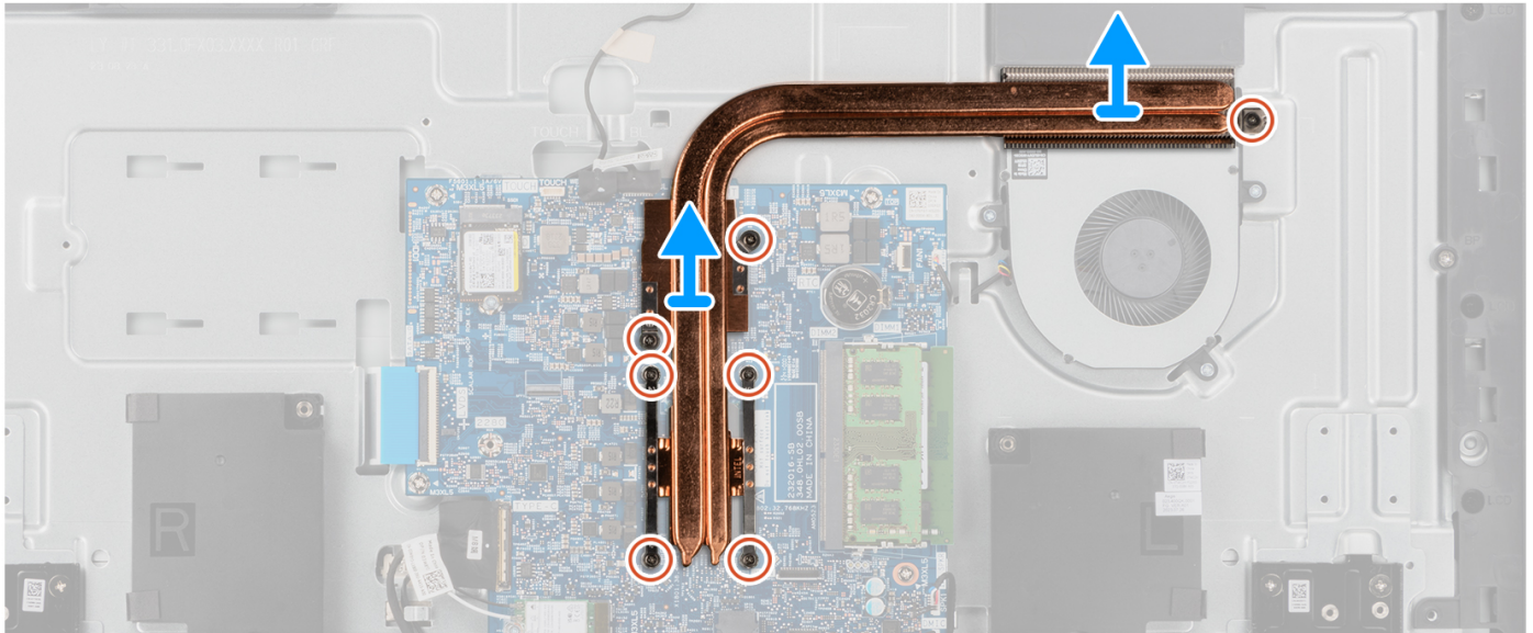
Figure 42. Removing the heat sink- UMA
