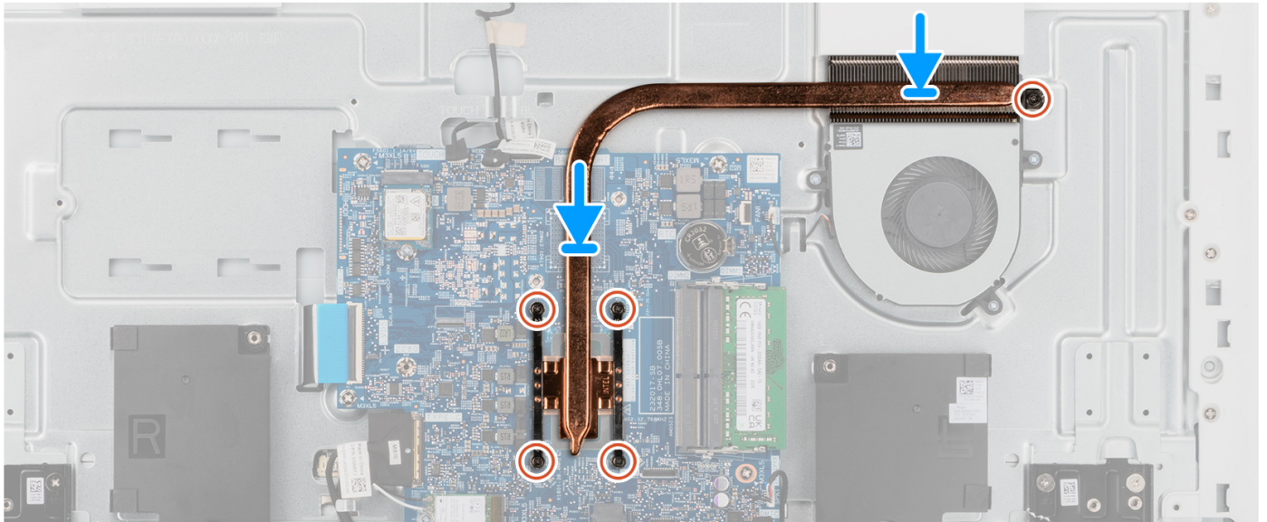
Figure 43. Installing the heat sink- UMA
