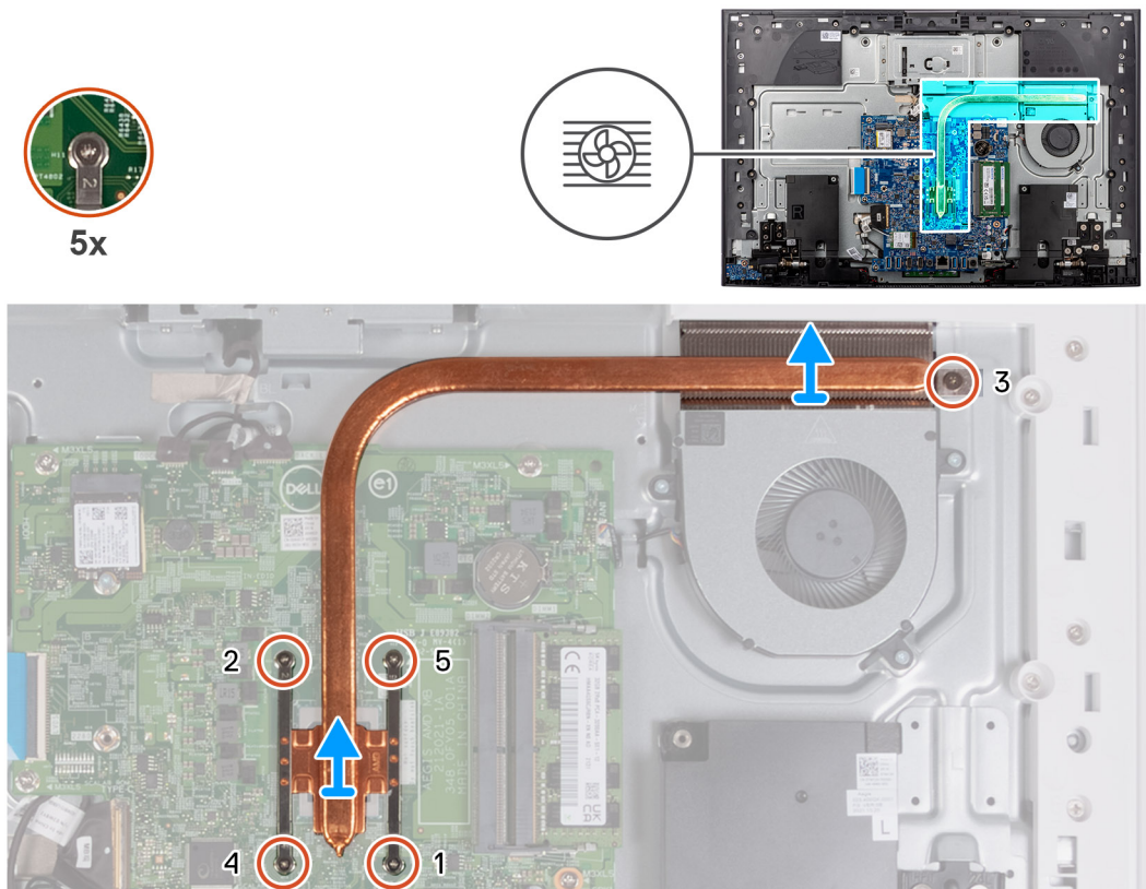
Figure 42. Removing the heat sink- UMA
