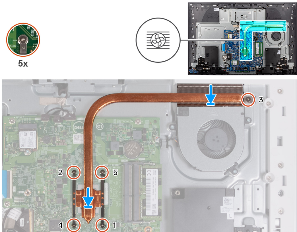
Figure 43. Installing the heat sink- UMA
